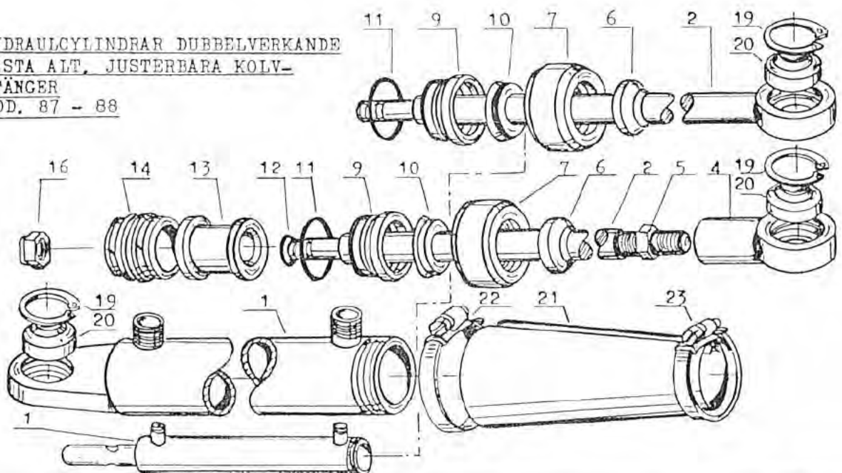
HYDRAULCYLINDRAR DUBBELVERKANDE MED GENOMGÅENDE KOLVSTÅNG MOD. 87 - 88
