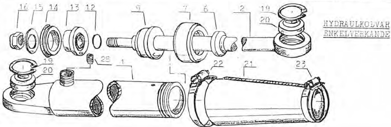
HYDRAULKOLVAR DUBBELVERKANDE FASTA ALT. JUSTERBARA KOLV- STÄNGER.
