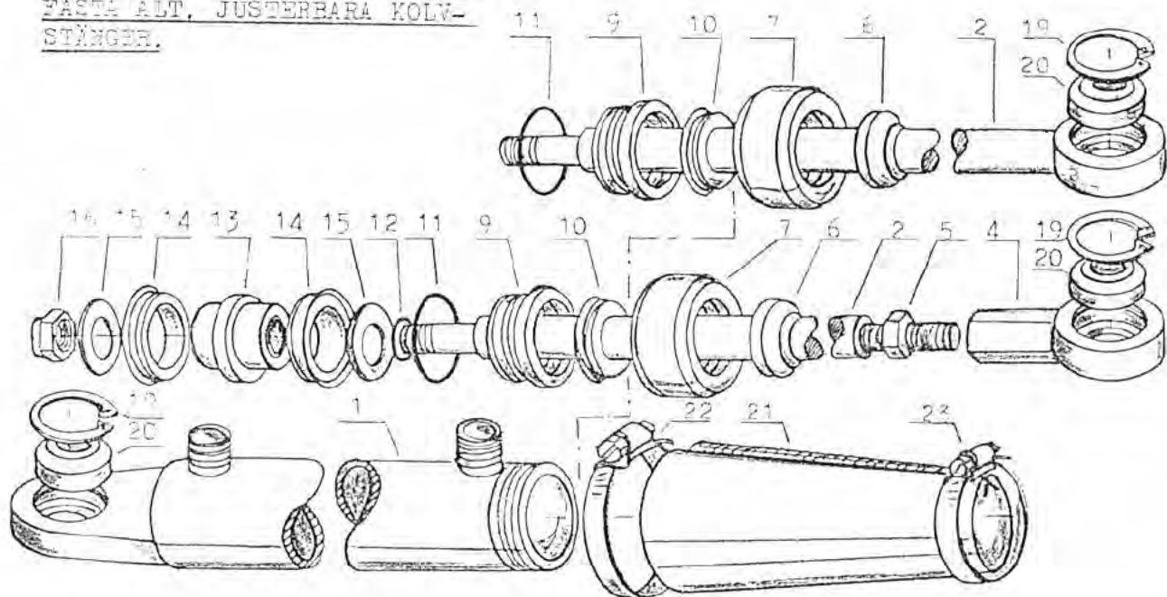
HYDRAULKOLVAR DUBBELVERKANDE MED GENOMGÅENDE KOLVSTANG.
