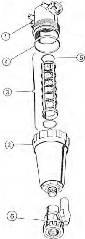
170 170 1 1/4" Tryckfilter med avtappning.
