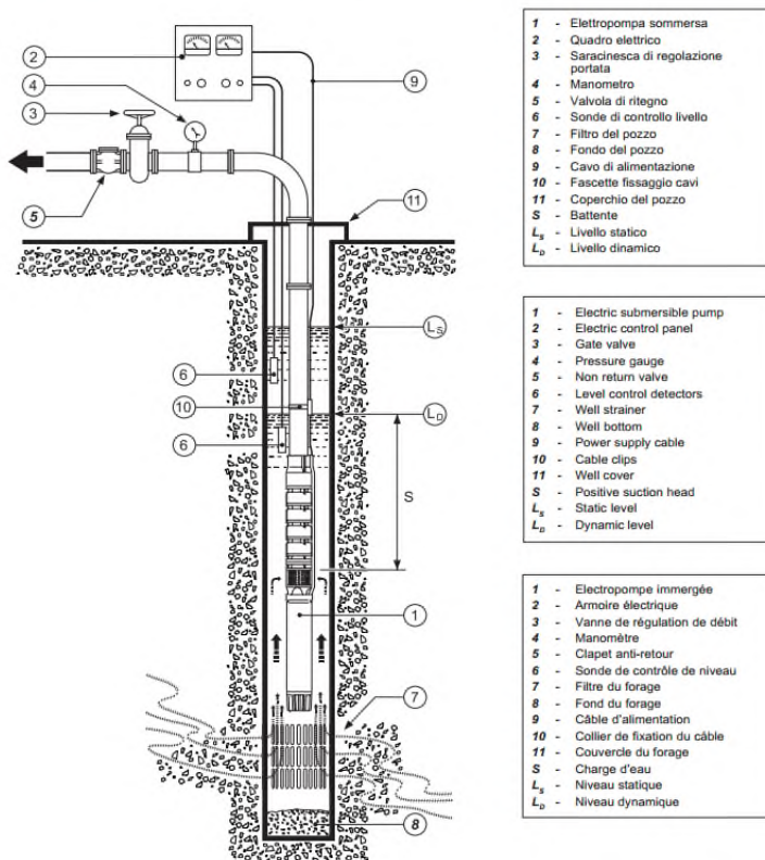
Schema installazione in pozzo - Well installation diagram - Schéma d'installation dans un forage
