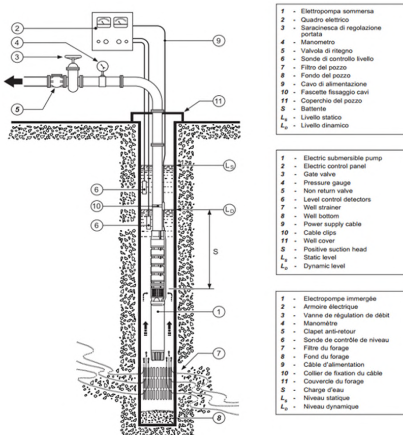
Schema installazione in pozzo - Well installation diagram - Schéma d'installation dans un forage
